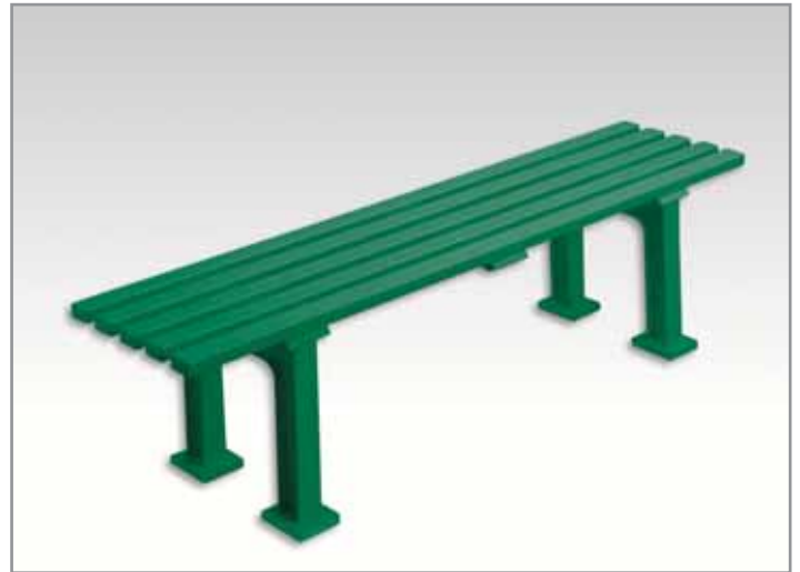
Bank München 150 cm Länge, grün 2 Vollkunststoff-FüÙe, sowie 5 Mehrkammerprofil-Latten, ohne Lehne daher beidseitig verwendbar, hoher Sitzkomfort. Gewicht ca. 9 kg. Nr. 412211 grün Stück € 107,60
