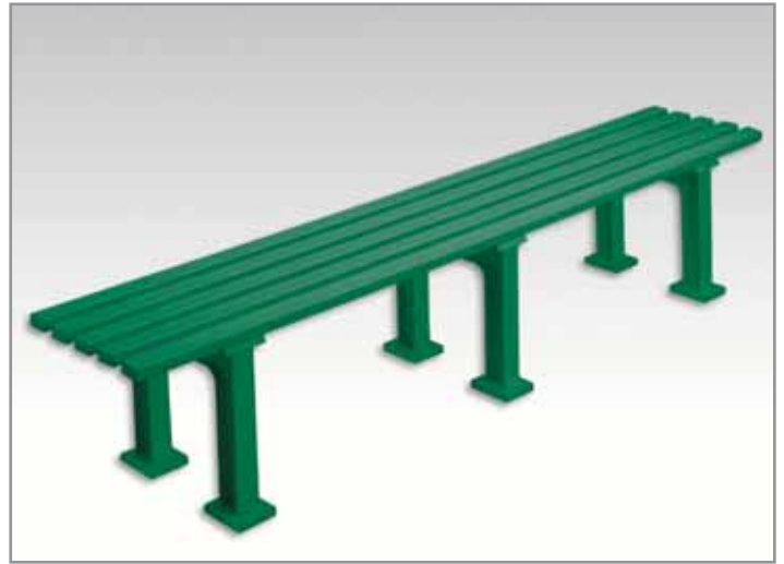
Bank Stuttgart 200 cm Länge, grün 3 Vollkunststoff-Füße, sowie 5 Mehrkammerprofil-Latten, ohne Lehne daher beidseitig verwendbar, hoher Sitzkomfort. Gewicht ca. 11,5 kg. Nr. 412213 grün
